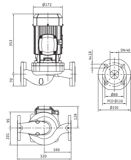
외형도(IL-I40/135-1.5/2)
